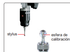
sonda (opcional), incluye palpador de Ø2mm y Ø3mm, esfera de calibración de Ø25mm y Ø3mm, la precisión de medición es de 10µm
