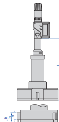
Tipo C 50-150mm, barra de medición de tres puntos de carburo
